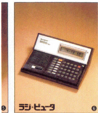
7 ラジ・セータ 情報先取りのラジオつき電卓 CT-610 ¥24,800 (デスクトップタイプ) ●AMラジオ(デジタルチューニング方式) ●タイマー機能 ●スリープ機能 ●連続使用約40時間(単2×3、ラジオのみ)
